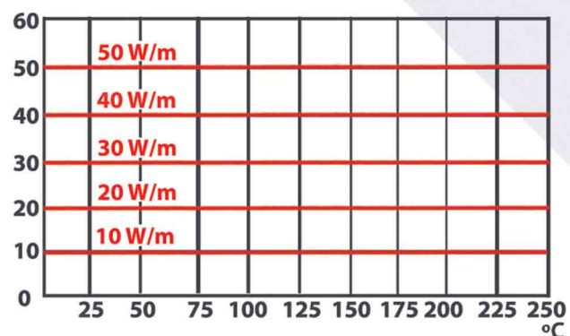
W/m Potência de acordo com a temperatura da tubulação
